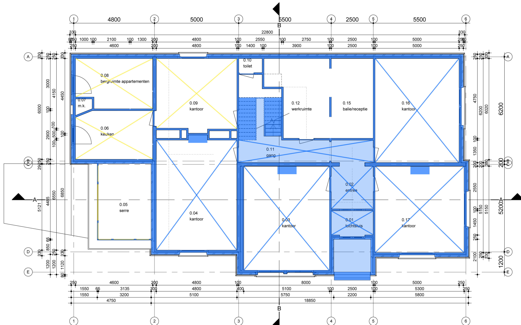
Begane grond
